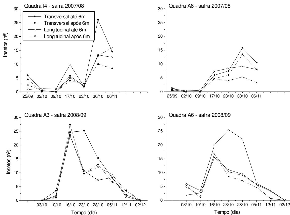
Figura 3. Flutuação populacional de adultos de O. oryzae (número médio de insetos por ponto amostral de acordo com a distância e orientação do caminhamento), em Itajaí, SC. Safra 2007/08 e 2008/09.
