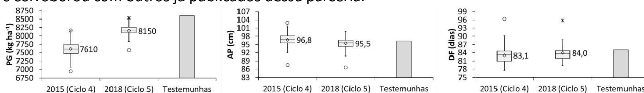
Figura 1. Boxplots de médias individuais (BLUP) de progênies de cada ciclo; e médias de tipos (BLUE de progênies de cada ciclo e de testemunhas), para os caracteres produtividade de grãos (PG), altura de plantas (AP) e dias para o florescimento (DF).
